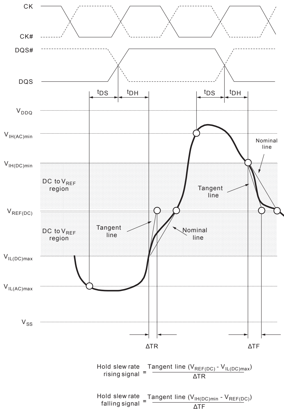
Figure 28 : Tangent Line for t DH (DQ – Strobe)
