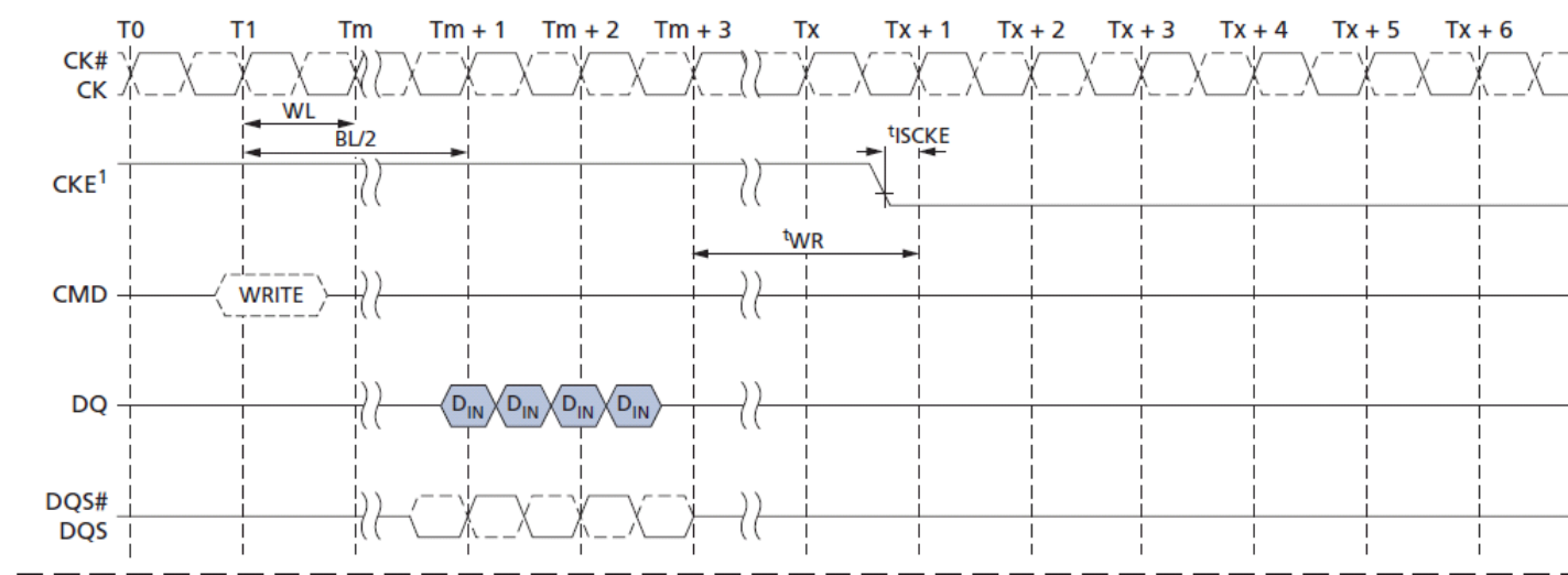
BL = 4
