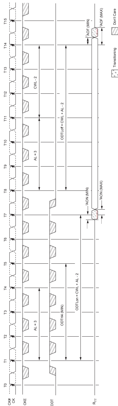
Figure 102 : Synchronous ODT
