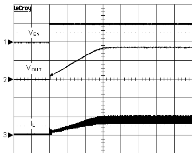
Enable
