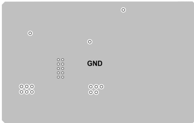
Inner Layer 2
