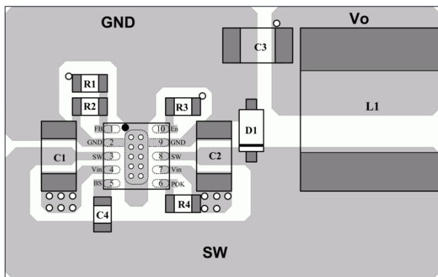
Top Layer
