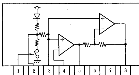
NJM2135L
